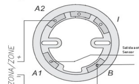
Diagrama de conexión de base de 2 hilos
