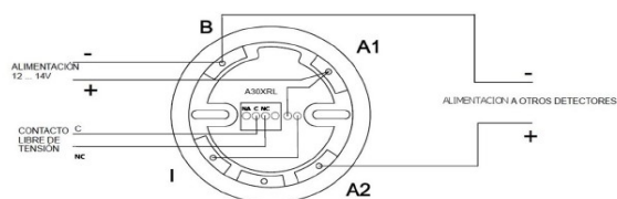
Diagrama de conexión de base de 4 hilos
