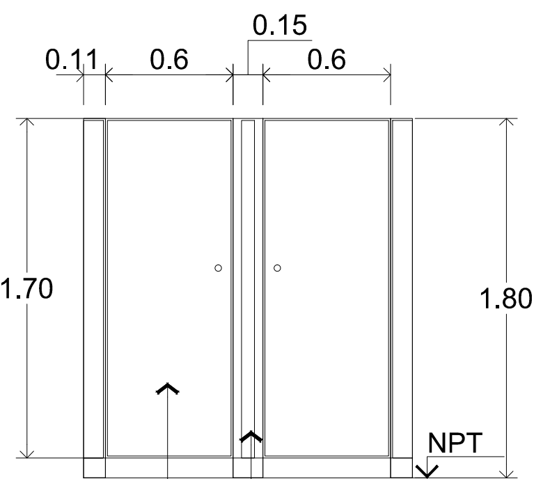
Panel tipo WC WALL Puerta de 0.60x1.70 m color a definir por la U.E.P.A.
