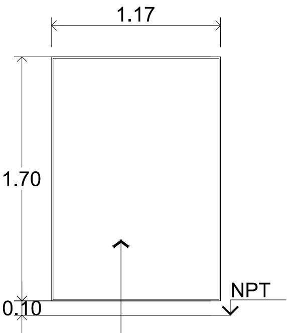
Panel lateral tipo WC WALL de 1.20x1.70 m color a definir
