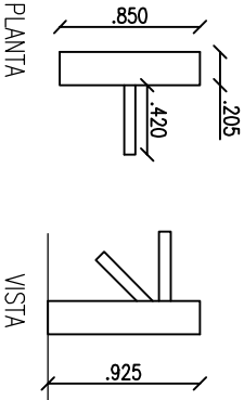
MOLINETE ESC: 1:50
